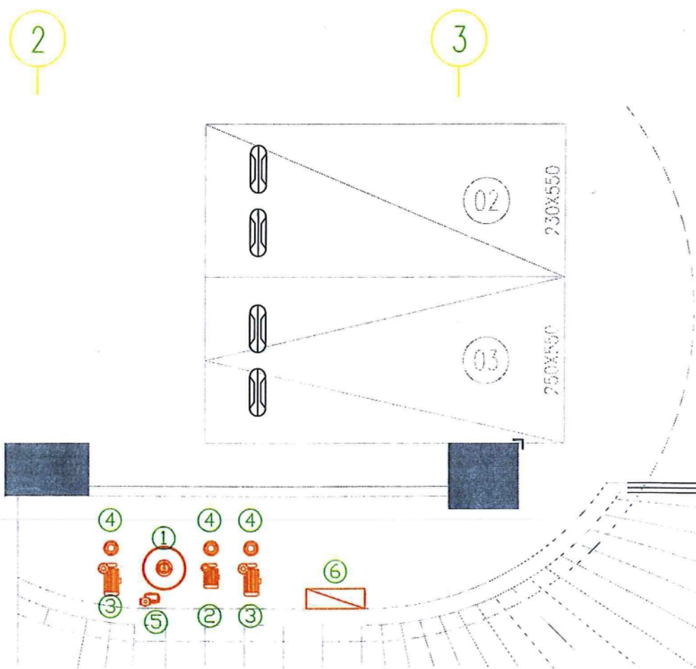
B1F 景觀機房配置平面圖
